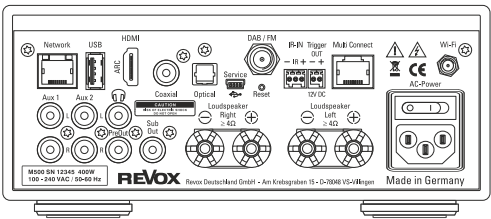
Rückansicht M300
